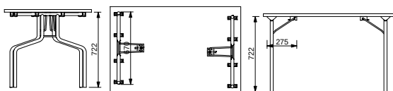
Hide chiuso - closed Versione - version (1200-1400) x 800 mm
