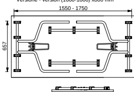
Hide chiuso - closed Versione - version (1600-1800) x 800 mm
