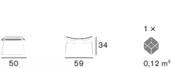
Nuvò 2005 POUF B200 Dimensioni / Sizes
