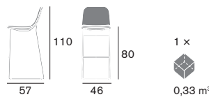
Nuvò 2005 SG 80 B302A Dimeansioni / Sizes
