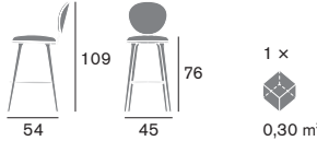
Giria 153 SG Dimensioni / Sizes
